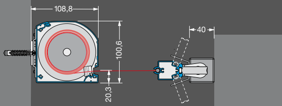
Befestigung mit Wandhalter [Standard] Draufsicht
