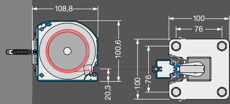
Befestigung mit Mast [Zusatzausstattung] Draufsicht
