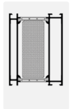
+ Rahmenverbreiterung | 100 mm
