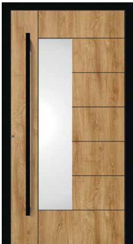
SILVA 1 - links | verglast Rahmenfarbe Schwarz RAL9005 Feinstruktur Türblatt turner oak malt senkrecht - Griffbereich senkrecht - Glas Satinato Weiß Stoßgriff Halbkreis-Formrohr 1600mm Schwarz Lisenen Planflächig Schwarz
